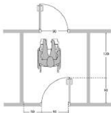
Schema dimensioni minime doppia porta consecutiva
